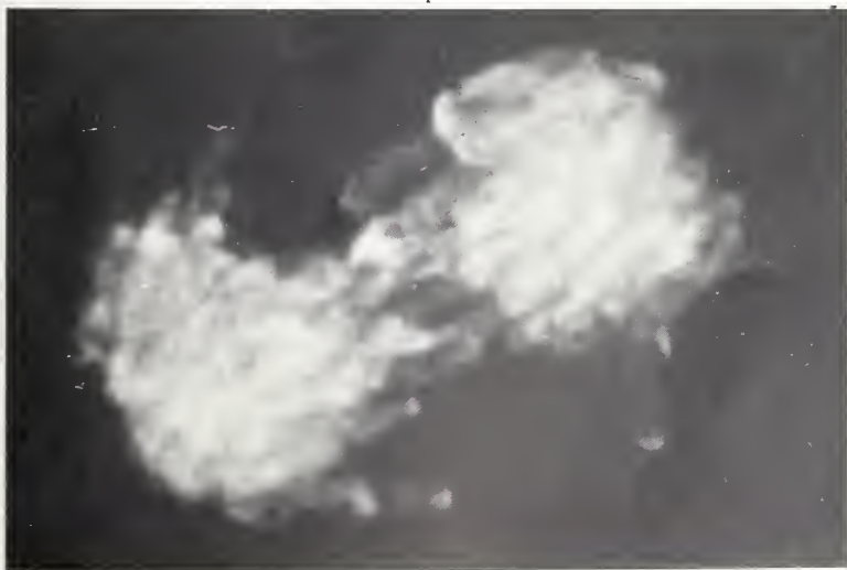
FIG. 8. Anaphase.
